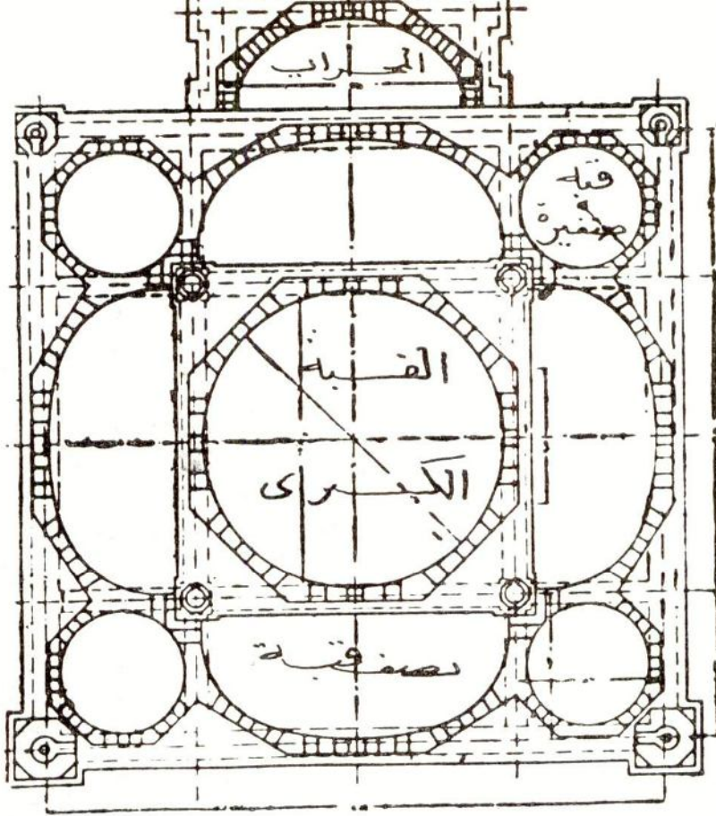
ش ٢ مسقط أفق للقسم الشرق وفيه قطاعات النوافذ
